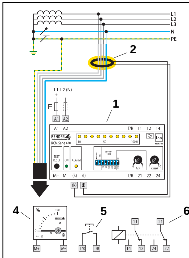
Anschluss Schaltbild
