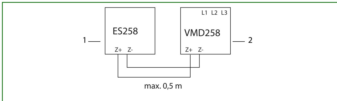
Abb. 2: Anschlussbild
